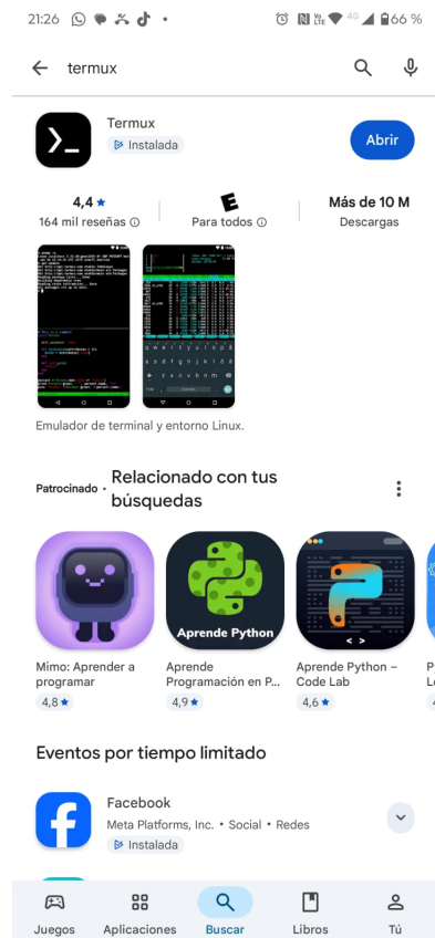
Figura 1: Termux
